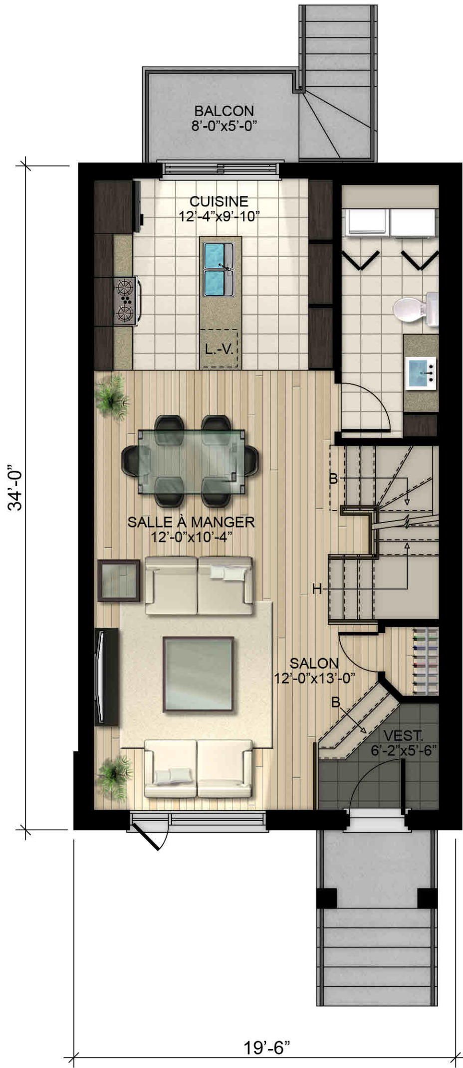
REZ-DE-CHAUSSÉE 654 pi 2
